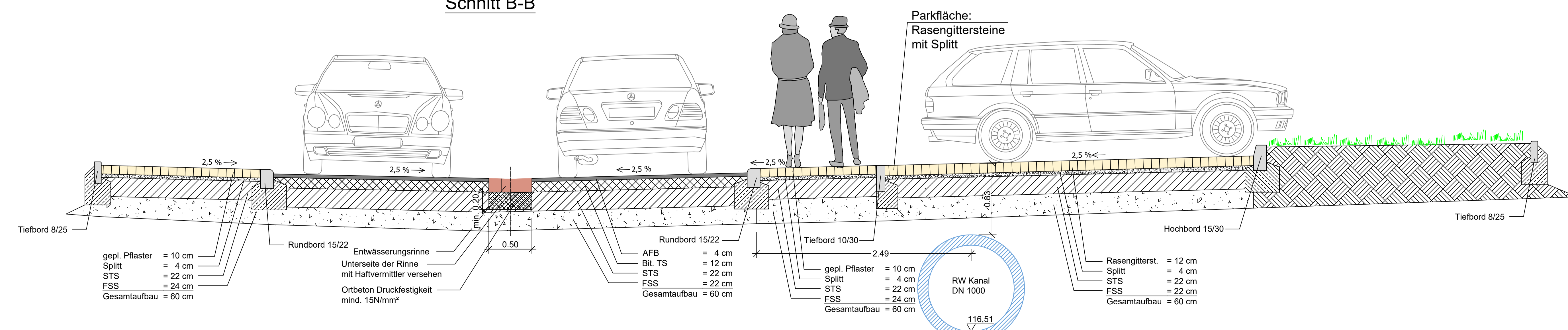
Schnitt B-B
