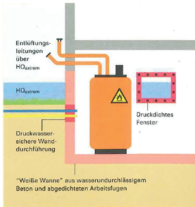
Heizöltanksicherung nach dem Prinzip „Wasser fernhalten“
