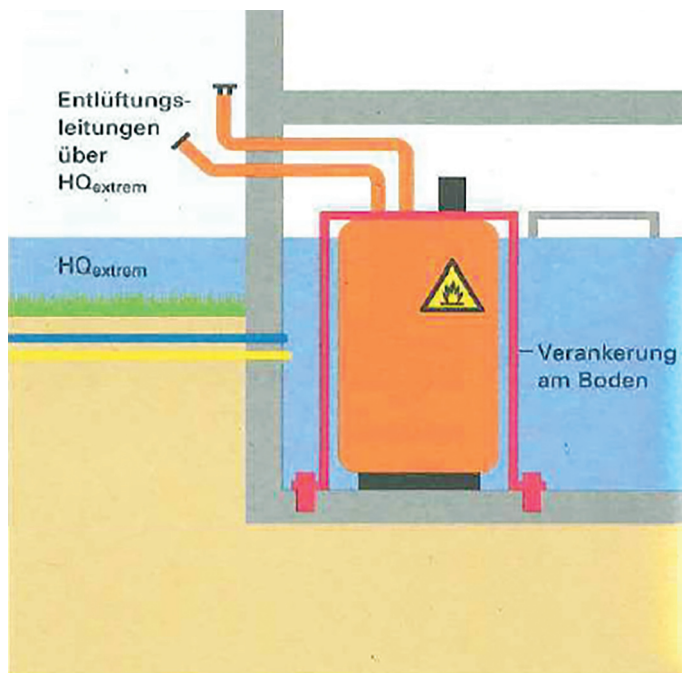
Heizöltanksicherung nach dem Prinzip „Anlagen sichern“
